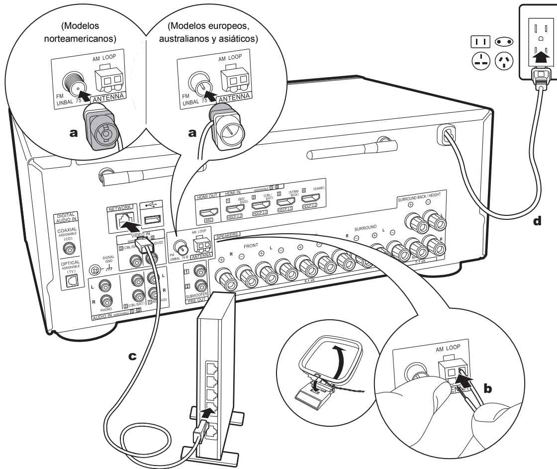
a Antena de FM para interiores, b Antena en bucle de AM, c Cable Ethernet, d Cable de alimentación
